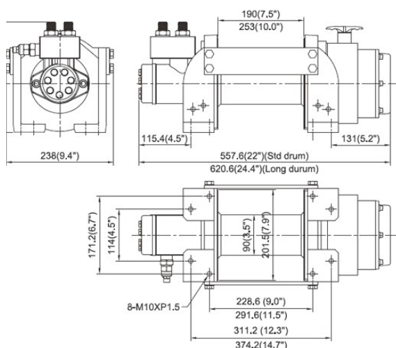
HV-8 & HV-8L mm/in
